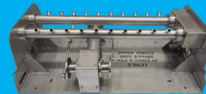
نازل بال پرنده Seagull swing nozzle
